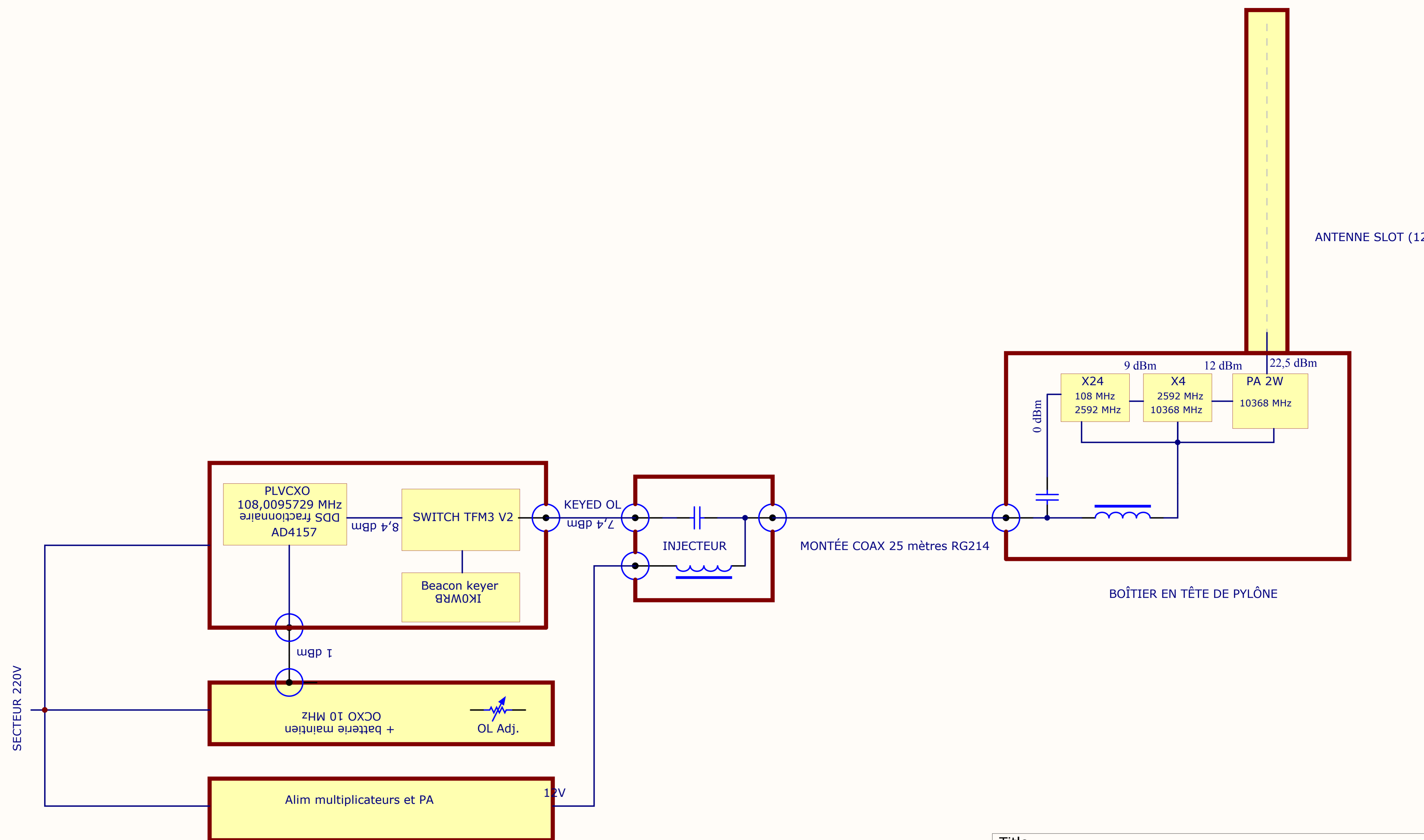
COFFRET ALIMENTATION, OXCO, PILOTE-KEYER, INJECTEUR DANS ABRI AU PIED DU PYLÔNE
