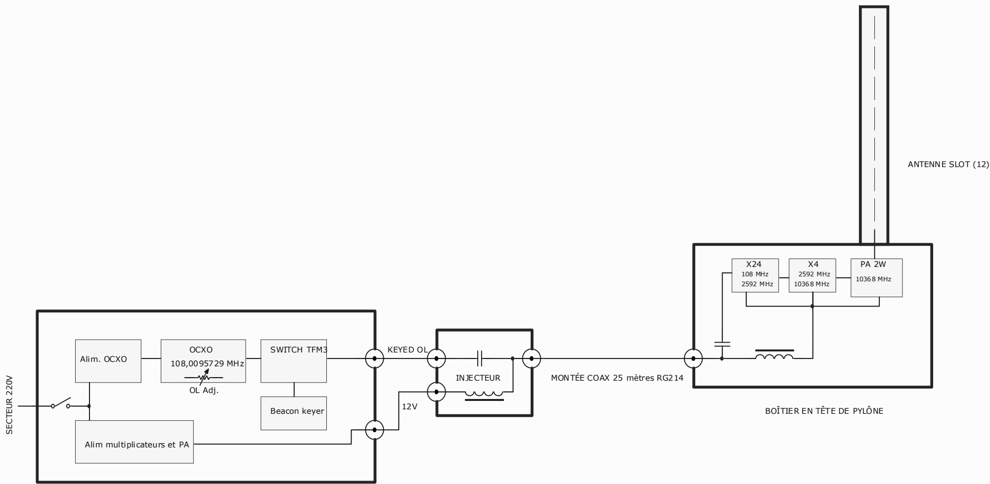
COFFRET ALIMENTATIONS, OL, MANIPULATION, INJECTEUR DANS ABRI AU PIED DU PYLÔNE
